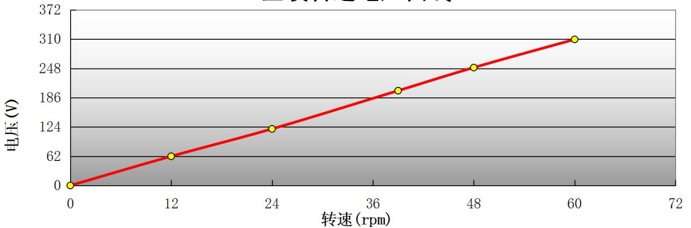
空载转速电压曲线
