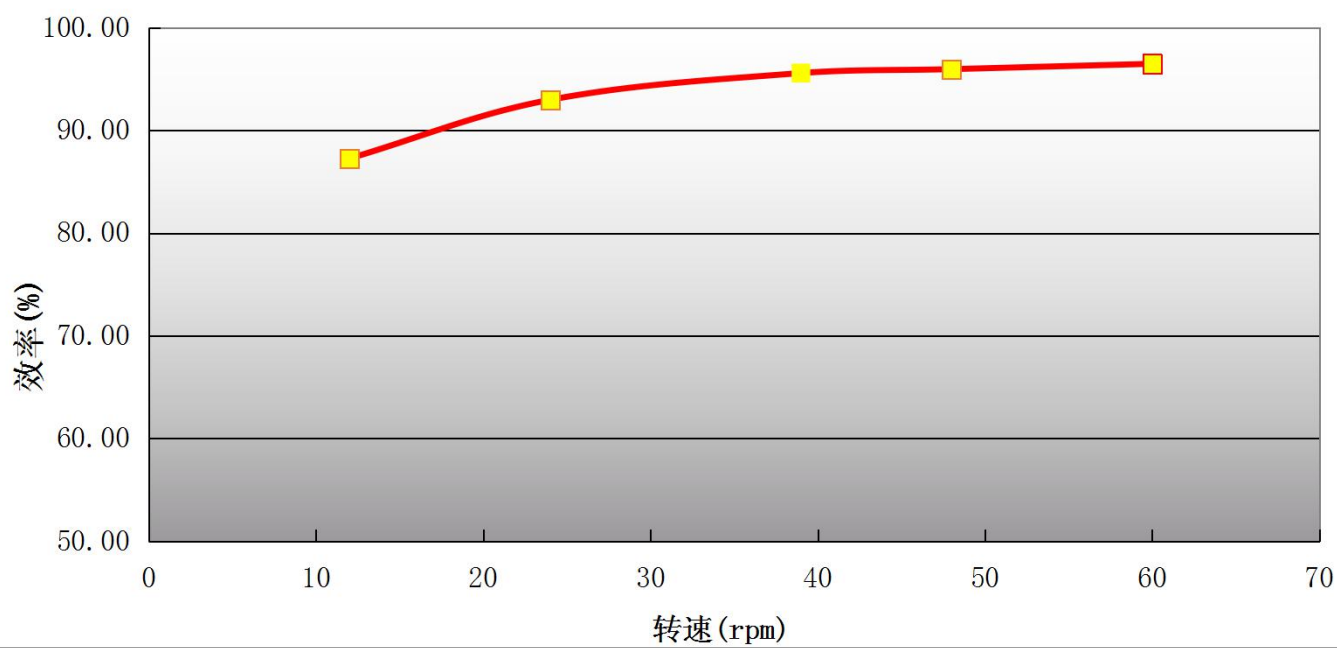
转速与效率曲线
