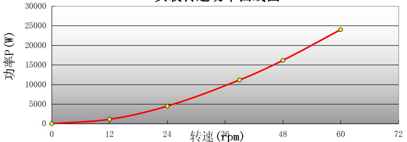
负载转速功率曲线图
