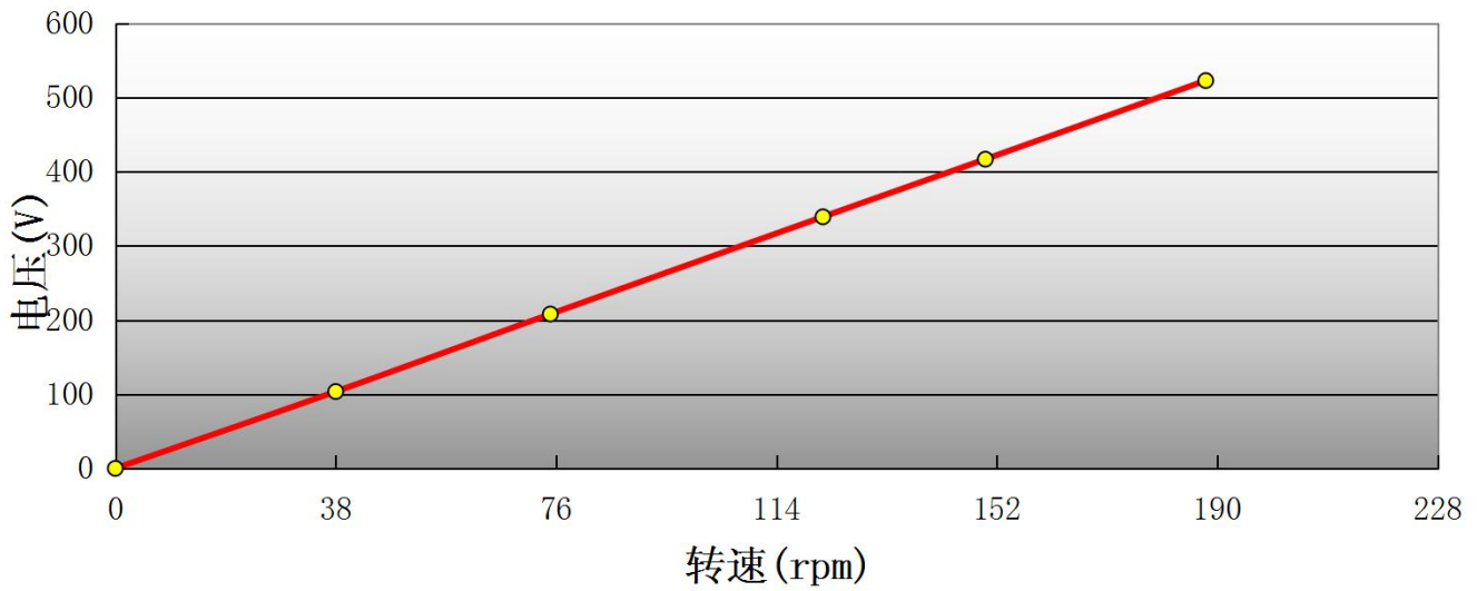
空载转速电压曲线
