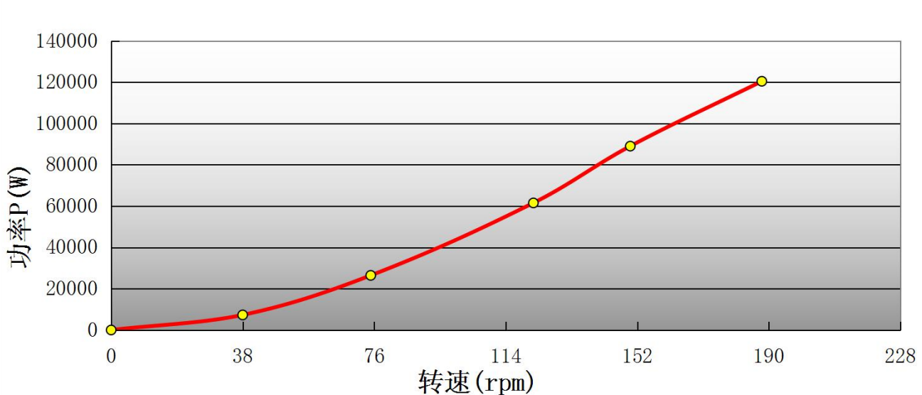
负载转速功率曲线图
