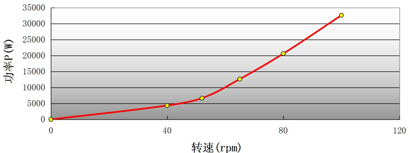
负载功率曲线图
