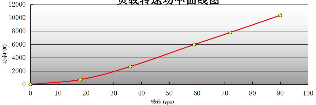
负载转速功率曲线图
