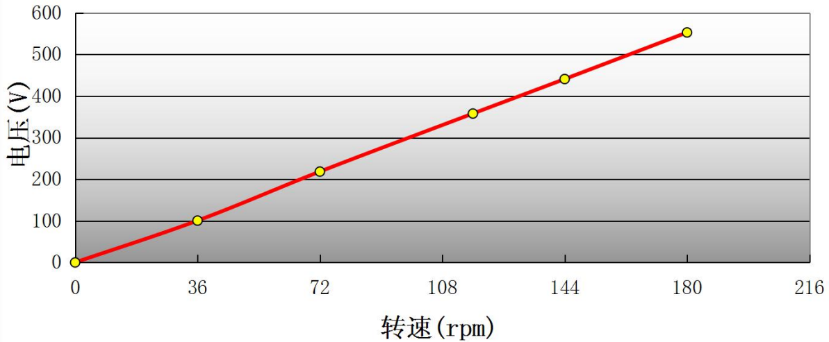
空载转速电压曲线
