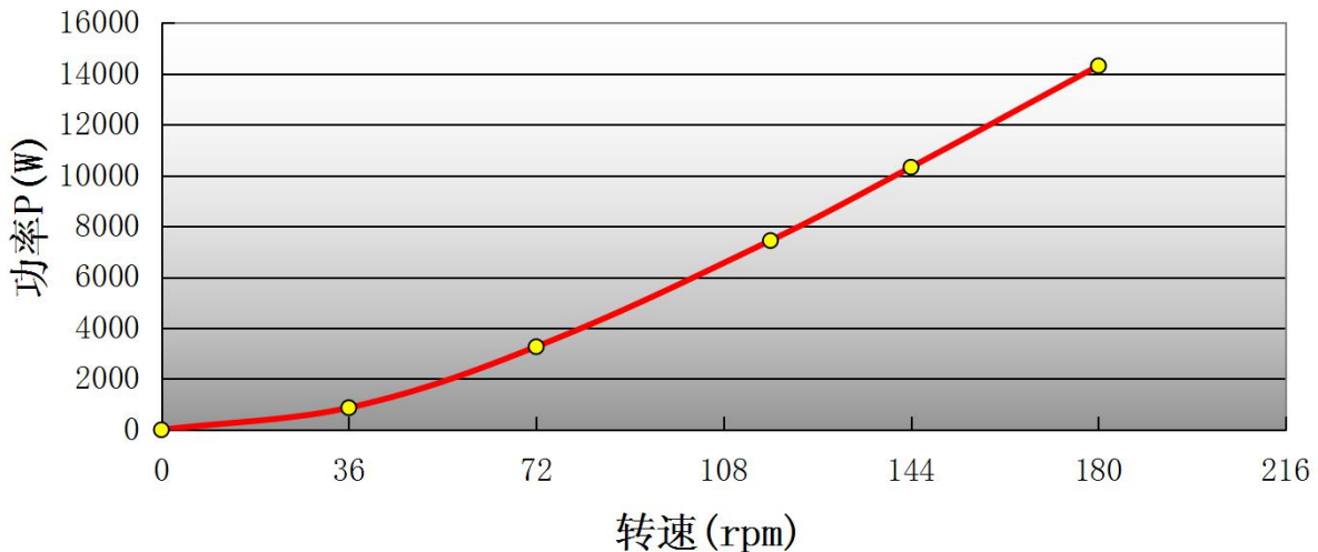
负载功率曲线图
