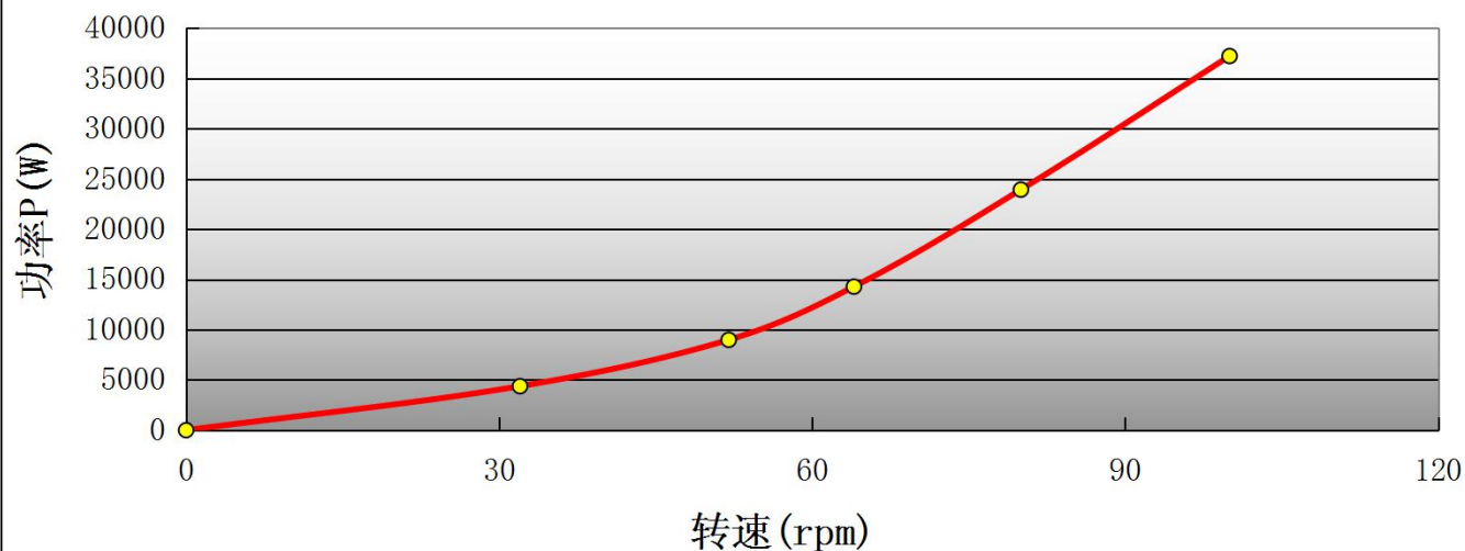
负载功率曲线图
