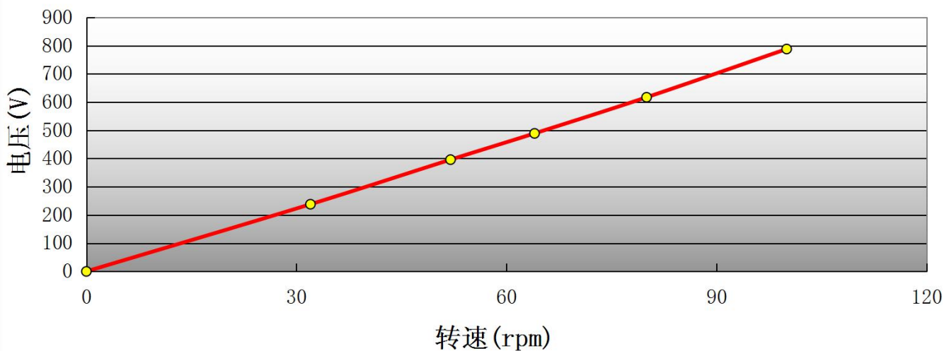
空载转速电压曲线
