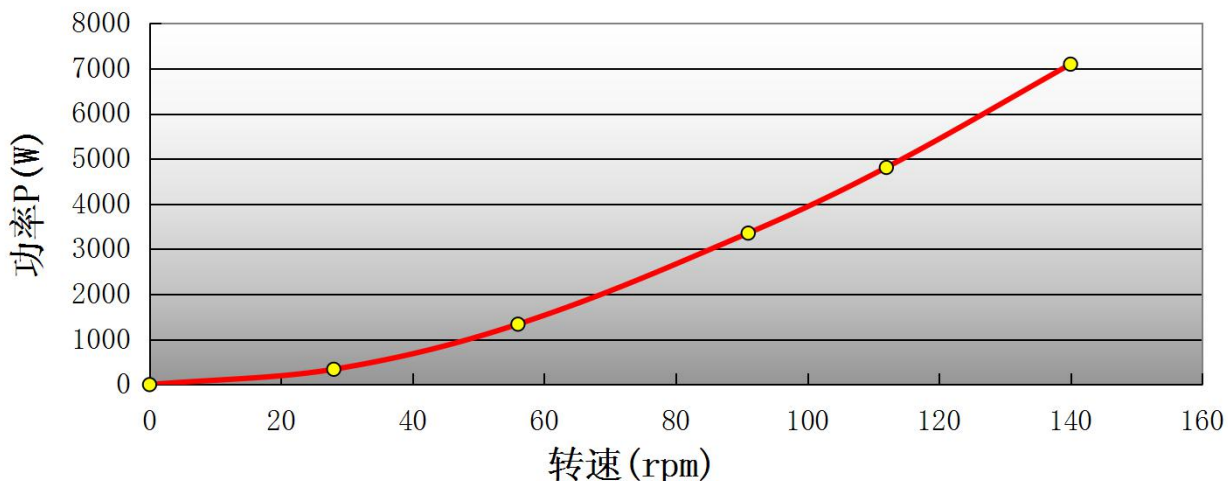
负载转速功率曲线图
