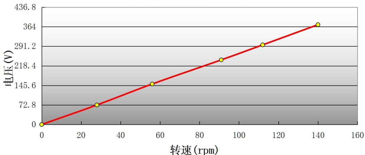
空载转速电压曲线
