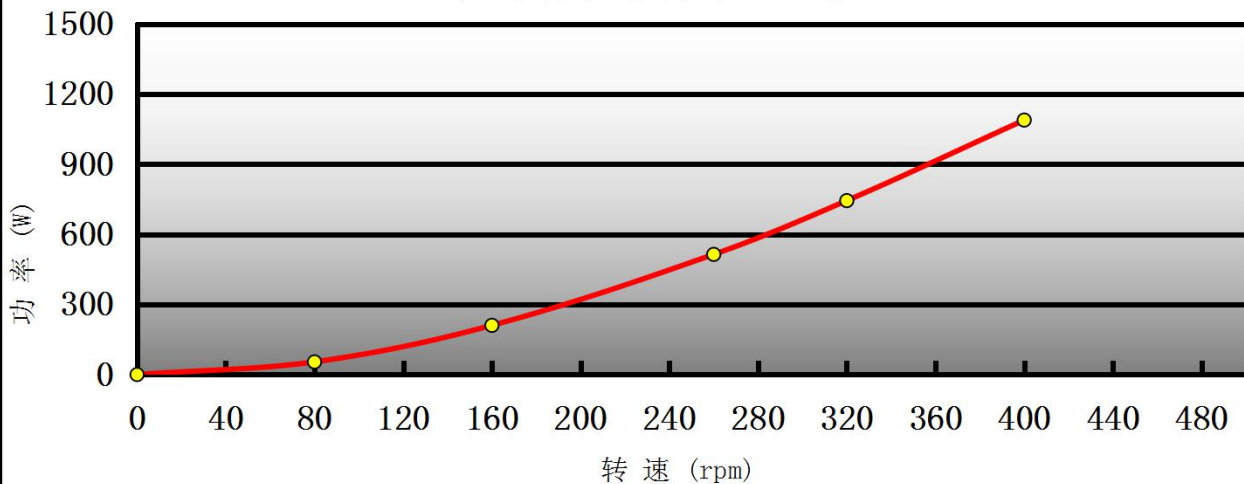
负载转速功率曲线
